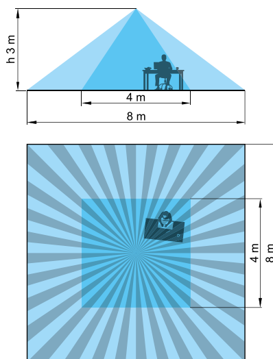
Sensor de presença e movimento
